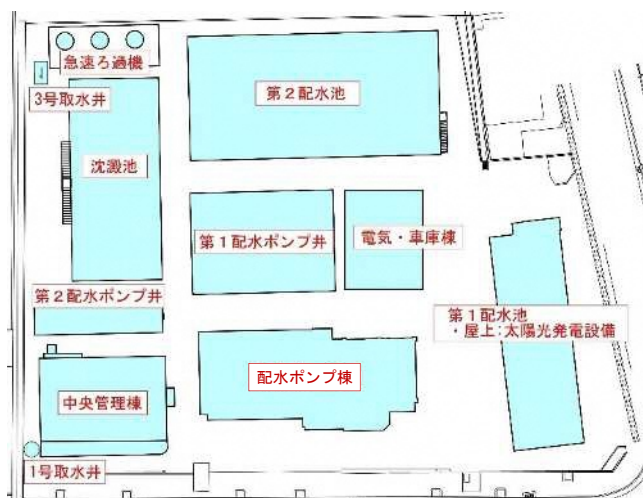
図 2.2 佐古浄水場
