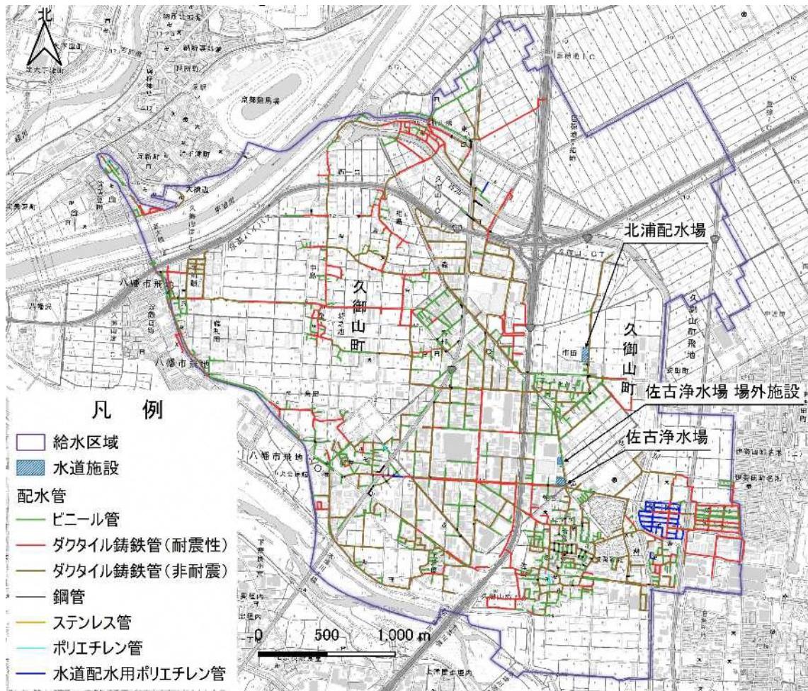
図 2.8 久御山町水道施設配置図 (令和 2 年度末)
